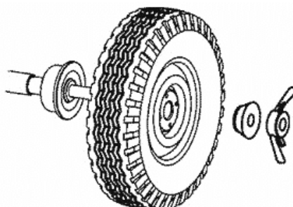
Рисунок 5.2 - Конус снаружи
