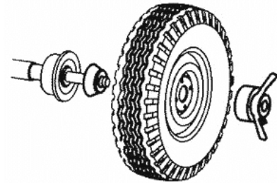
Рисунок 6.9 – Установка колеса
