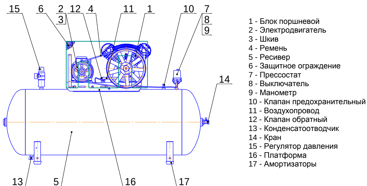
Рисунок 7 - Общий вид компрессоров СБ4/Φ-500.LB50-5.5
